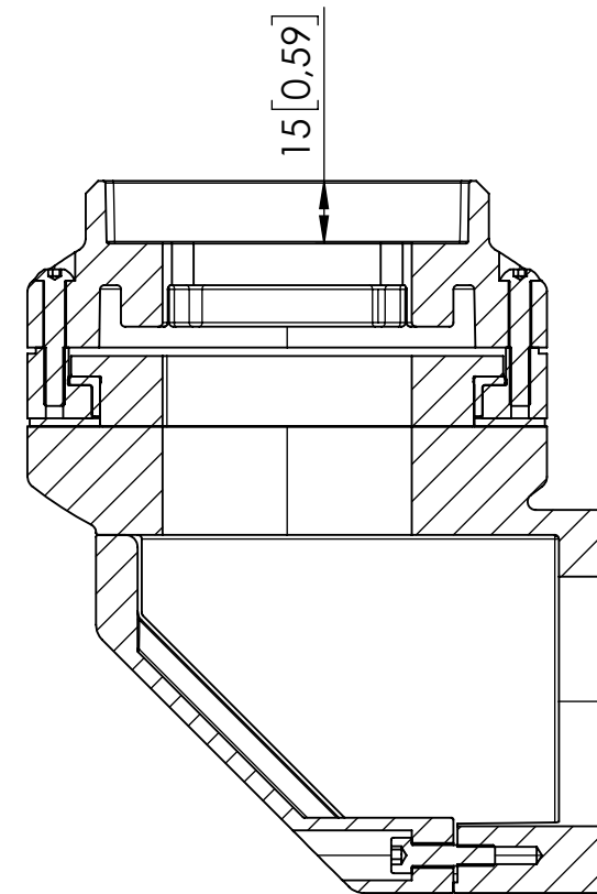
SCHNITT A-A
