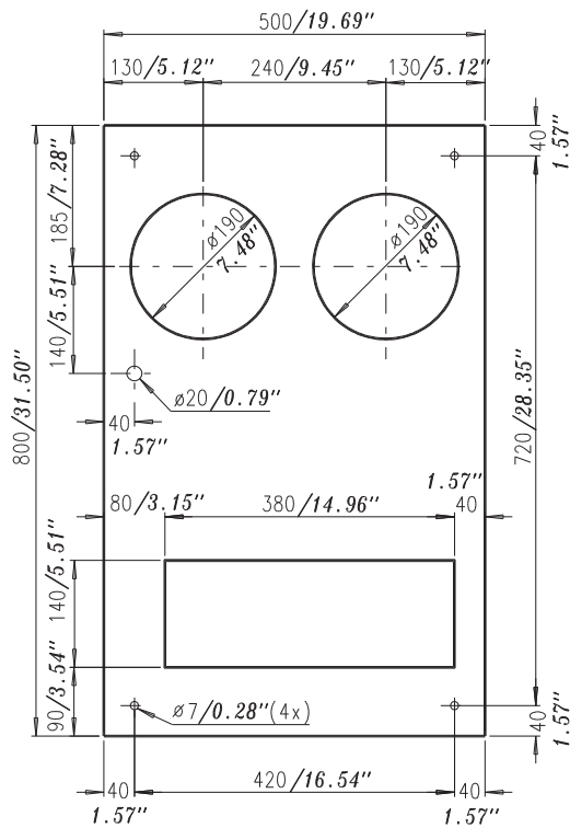
Lochbild Schrankanbau Drilling template external mounting Gabarit de perçage montage extérieur
