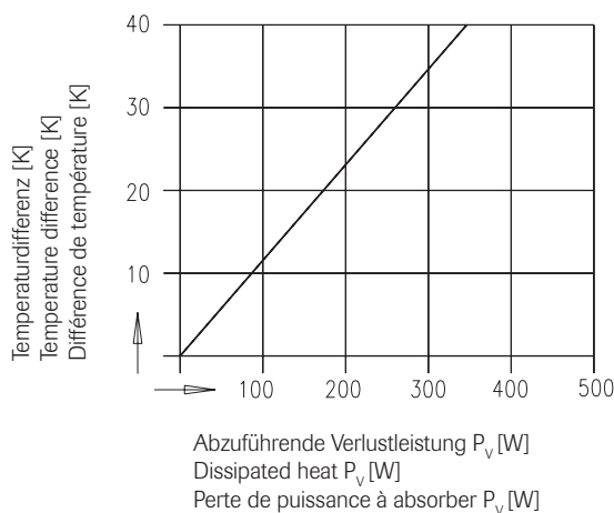
Leistungsdiagramm Performance diagram Diagramme de puissance
