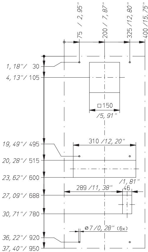
Lochbild Schrankanbau
