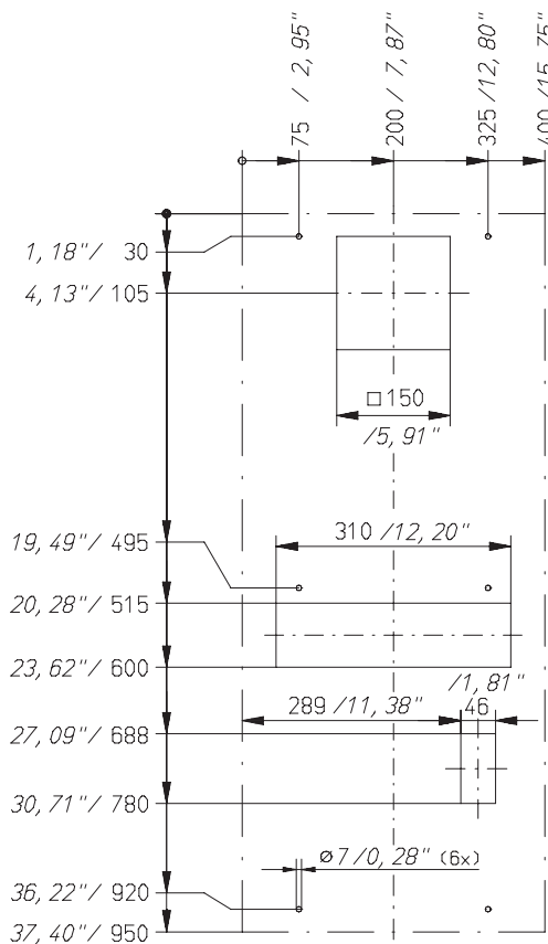
Gabarit de perçages montage extérieur
