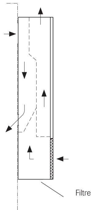
Circuit d'air et découpes
