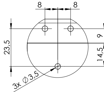
DETAIL A MABSTAB 1 : 1
