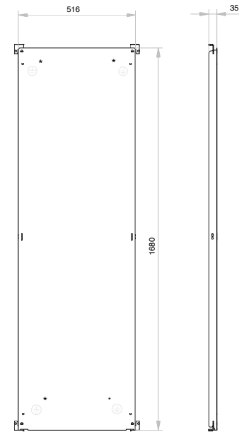
Montageplatte sendzimirverzinkt Blechstärke = 2,5 mm
