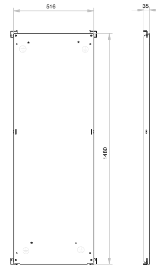
Montageplatte sendzimirverzinkt Blechstärke = 2,5 mm
