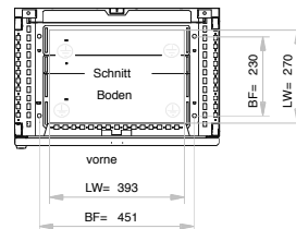
dreiteilige Bodenplatte frei einteilbar
