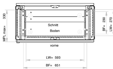
dreiteilige Bodenplatte frei einteilbar
