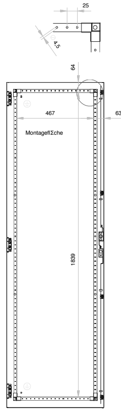
Türe Innenseite
