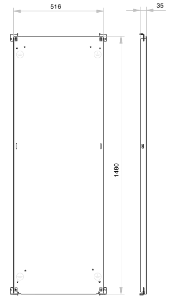
Montageplatte sendzimirverzinkt Blechstärke: 2,5 mm
