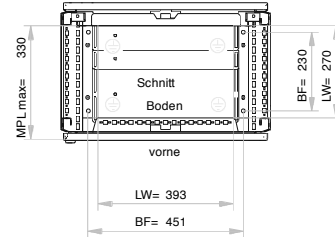
dreiteilige Bodenplatte frei einteilbar
