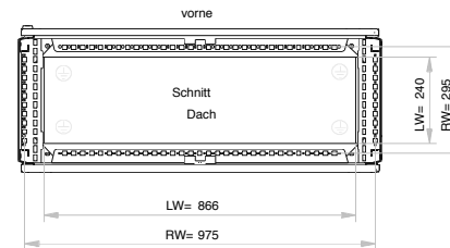
vorne
