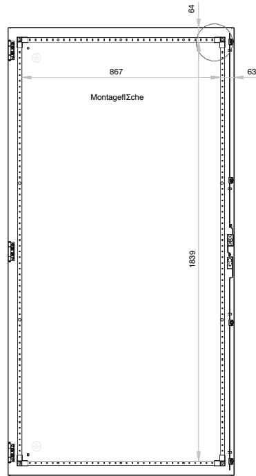
T're Innenseite
