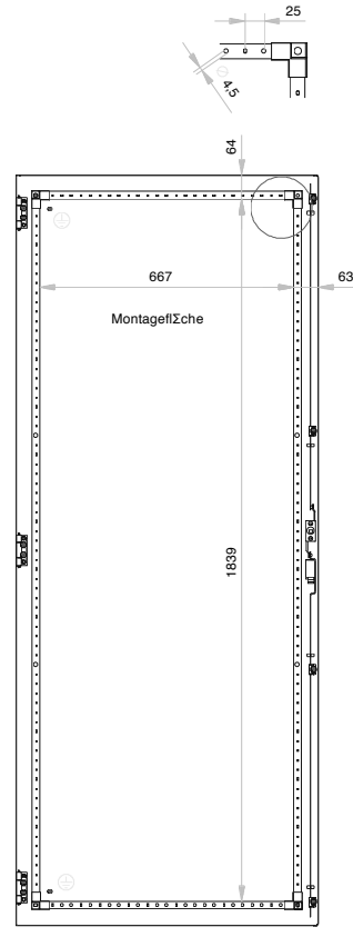
Türe Innenseite
