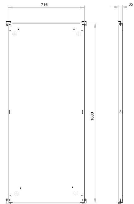
Montageplatte sendzimirverzinkt Blechstärke = 2.5 mm
