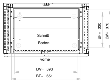
dreiteilige Bodenplatte frei einteilbar
