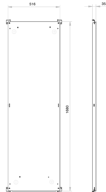
Montageplatte sendzimirverzinkt Blechstärke = 2,5 mm
