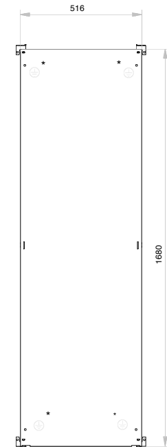
Montageplatte sendzimirverzinkt
