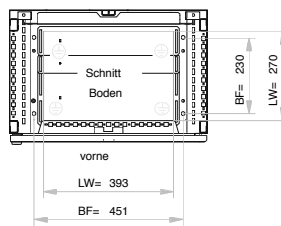
dreiteilige Bodenplatte frei einteilbar
