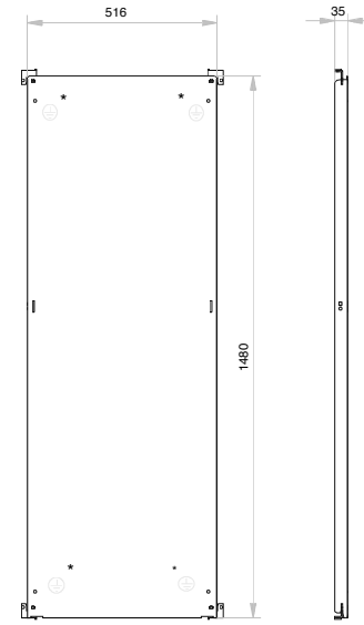
Montageplatte sendzimirverzinkt Blechstärke = 2,5 mm
