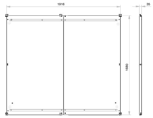
Montageplatte sendzimirzinkt Blechstärke = 3,0 mm
