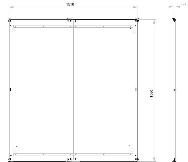
Montageplatte sendzimirverzinkt Blechstärke = 3,0 mm
