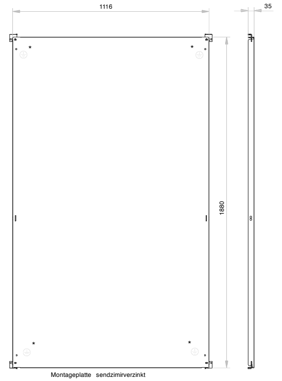
Montageplatte sendzimirverzinkt Blechstärke = 3,0 mm
