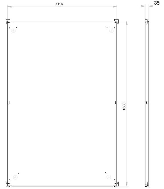
Montageplatte sendzimirverzinkt Blechst'zrke = 3,0 mm
