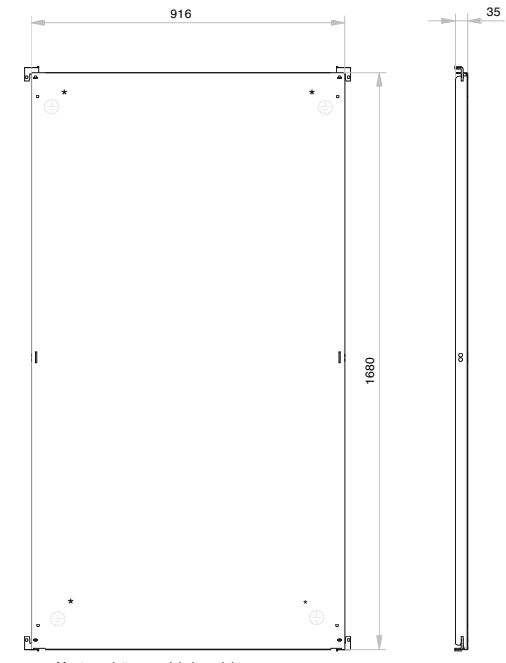
Montageplatte sendzimirzinkt Blechstärke = 3,0 mm
