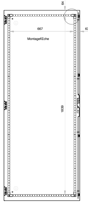
Türe Innenseite
