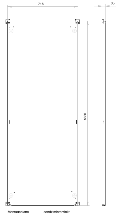
Montageplatte sendzimirzinkt Blechstärke: 2,5 mm
