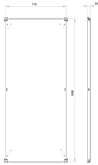
Montageplatte senkzimirverzinkt Blechstr'ke: 2,5 mm
