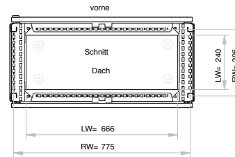
vorne
