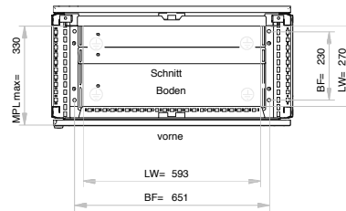
dreiteilige Bodenplatte frei einteilbar
