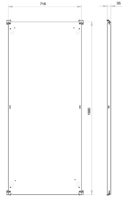
Montageplatte sendzimirverzinkt BlechStärke: 2,5 mm
