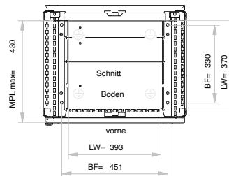
dreiteilige Bodenplatte frei einteilbar
