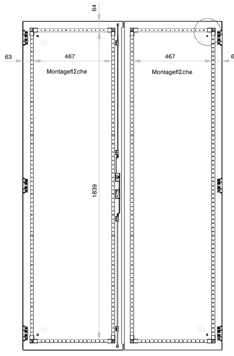
Türe Innenseite
