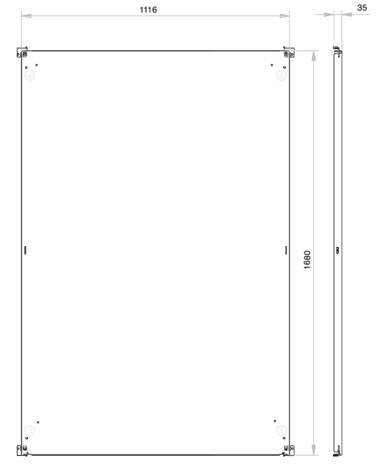
Montageplatte sendzimirzinkt Blechstrke: 3,0 mm
