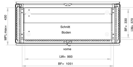
dreiteilige Bodenplatte frei einteilbar
