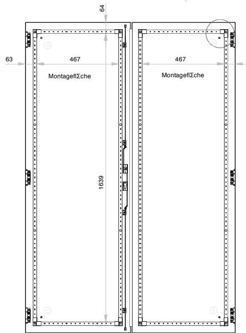
Tre Innenseite
