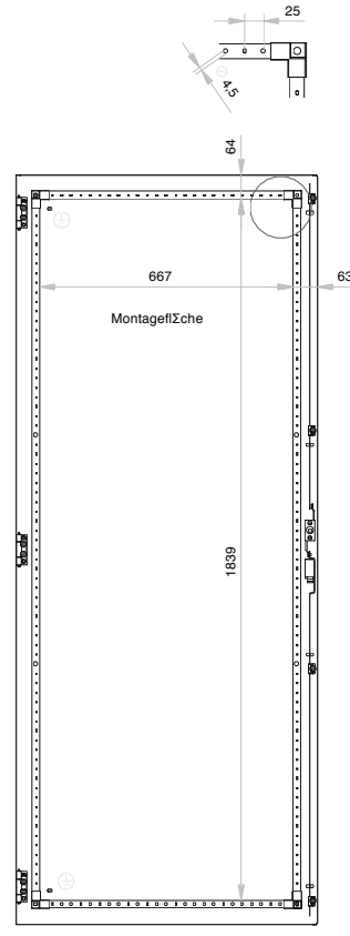
Türe Innenseite
