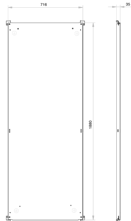
Montageplatte sendzimirverzinkt Blechstärke = 2,5 mm
