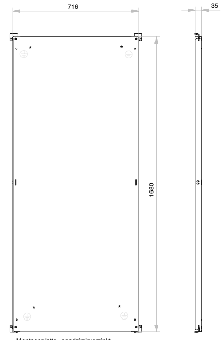
Montageplatte sendzimirverzinkt Blechstärke = 2,5 mm
