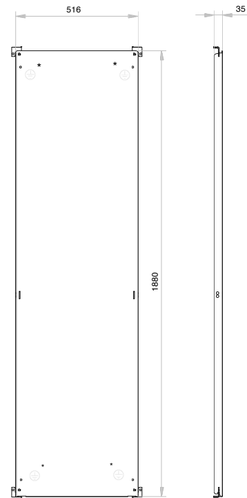
Montageplatte sendzimirverzinkt Blechstärke = 2,5 mm
