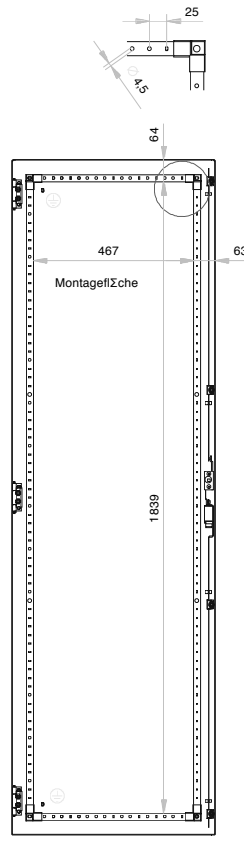
Türe Innenseite
