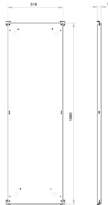
Montageplatte sendzimirverzinkt Blechst'rke = 2,5 mm
