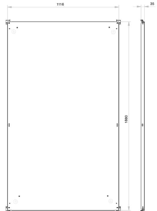
Montageplatte sendzimirzinkt Blechstärke = 3,0 mm
