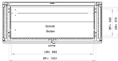
dreiteilige Bodenplatte frei einteilbar
