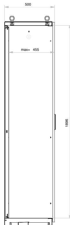
dreiteilige Bodenplatte frei einteilbar
