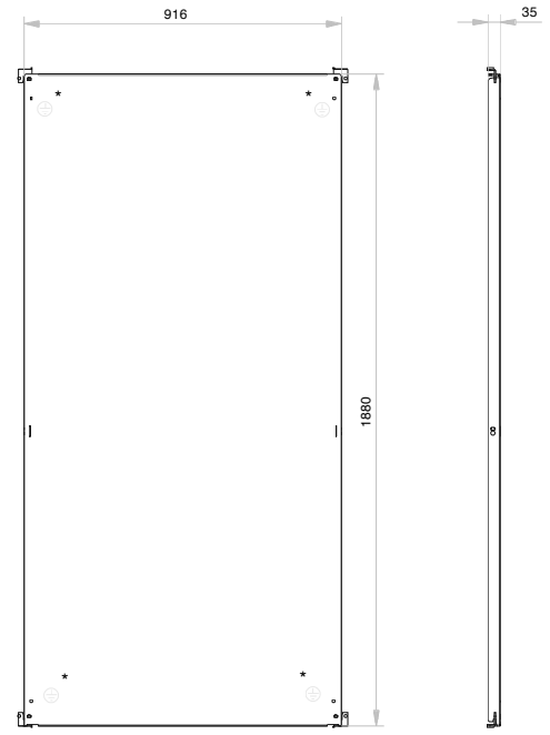
Montageplatte sendzimirverzinkt Blechst'zrke = 3,0 mm
