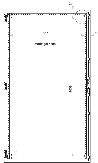
T're Innenseite
