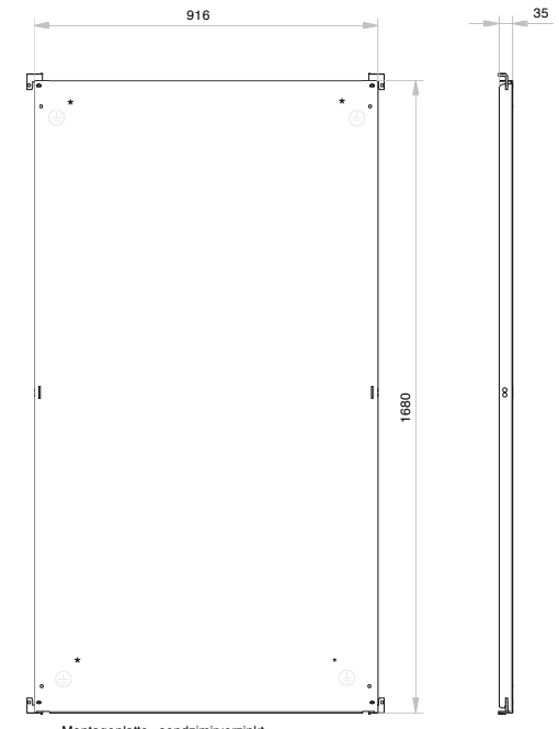
Montageplatte sendzimirzinkt
