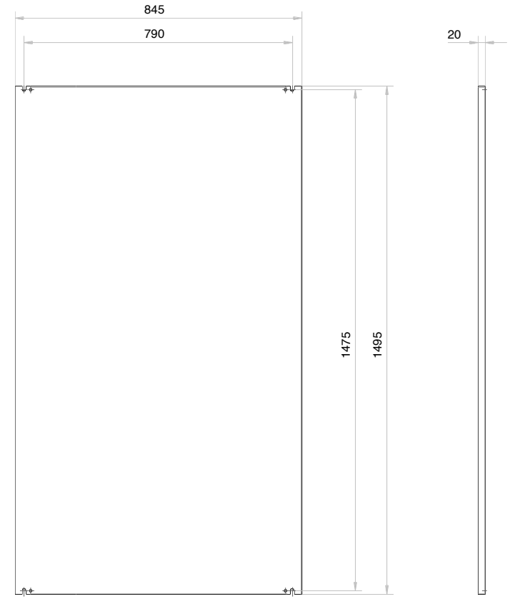
Einbauplatte sendzimirverzinkt
