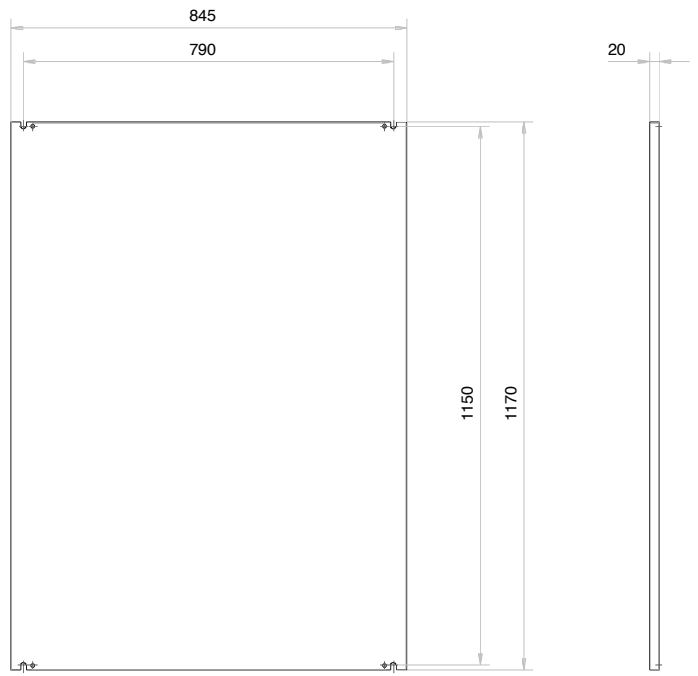
Einbauplatte sendzimirverzinkt
