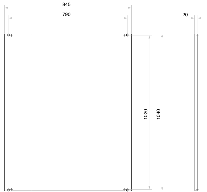
Einbauplatte sendzimirverzinkt
