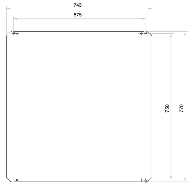
Einbauplatte sendzimirverzinkt
