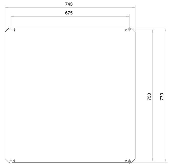
Einbauplatte sendzimirverzinkt
