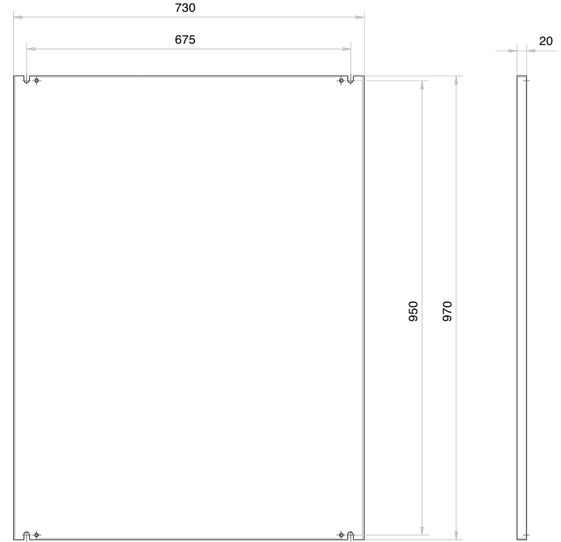
Einbauplatte sendzimirverzinkt
