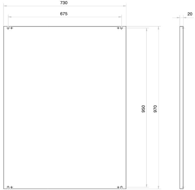
Einbauplatte sendzimerverzinkt
