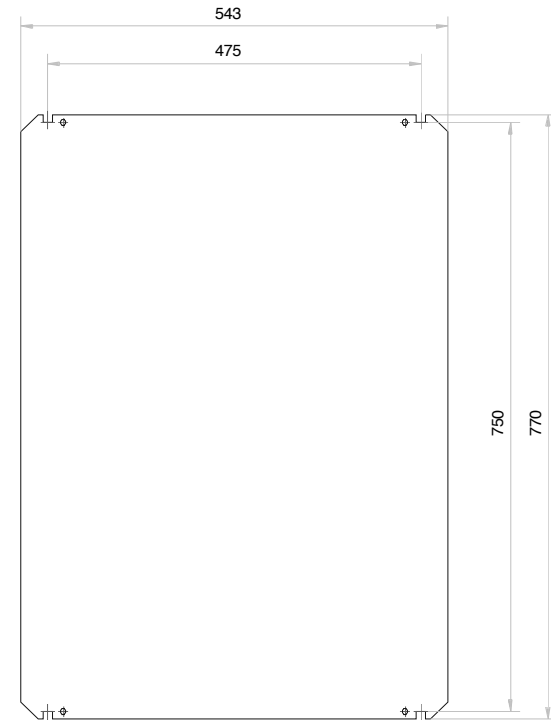
Einbauplatte sendzimirverzinkt
