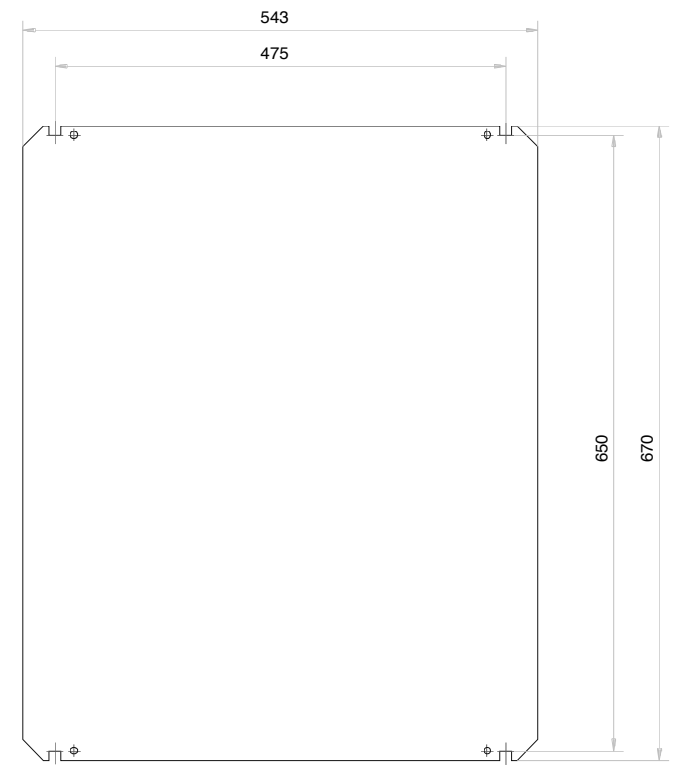
Einbauplatte sendzimirverzinkt
