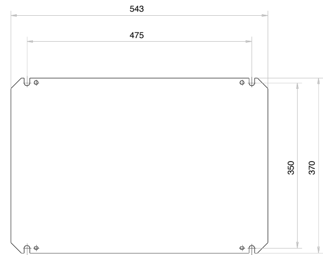
Einbauplatte sendzimirverzinkt
