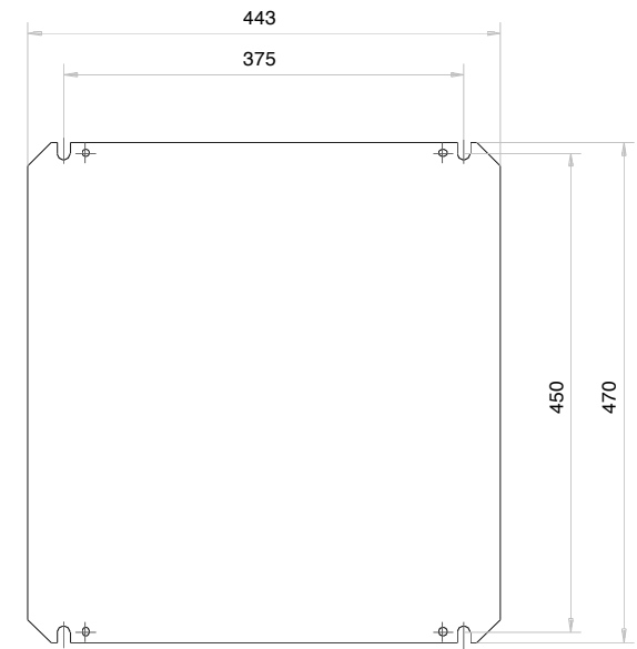
Einbauplatte sendzimirverzinkt
