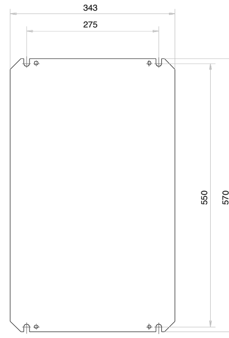
Einbauplatte sendzimirverzinkt
