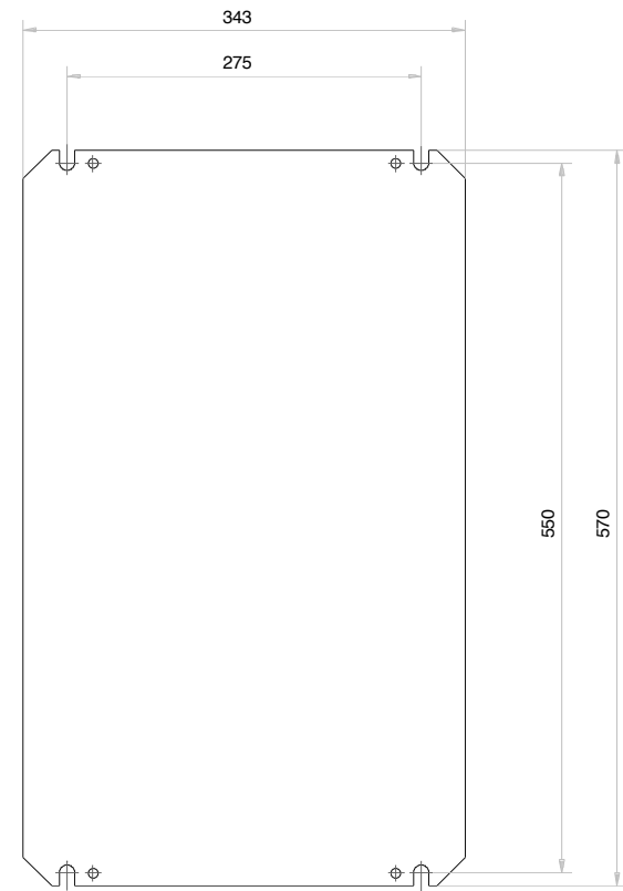
Einbauplatte sendzimirverzinkt
