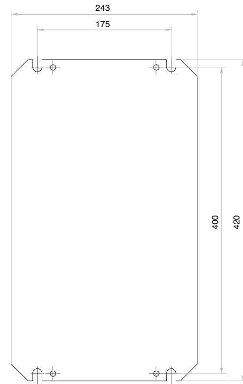
Einbauplatte sendzimirverzinkt
