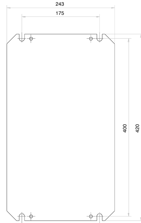
Einbauplate sendzimirverzinkt
