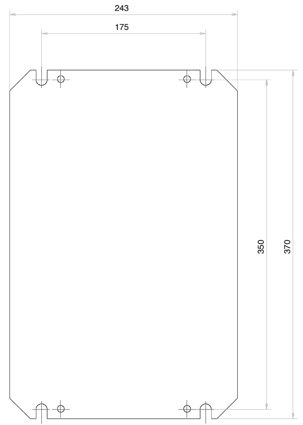
Einbauplatte sendzimirverzinkt
